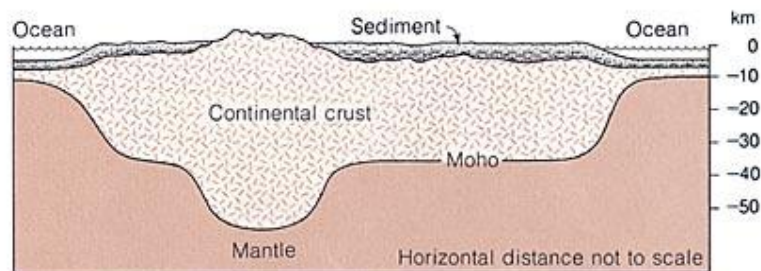
Figuur 7: De bergen hebben diepe wortelen in het grondoppervlak ( Earth , Press and Siever, p. 413)
