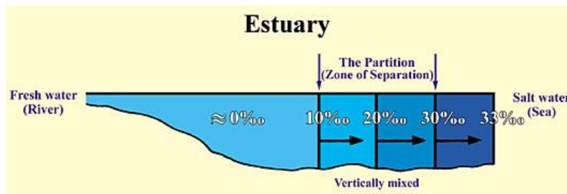
Figuur 14: Overlangse doorsnede van een estuarium laat de zoutdichtheid (gedeeltes zijn in promille (‰) weergegeven) zien. We kunnen hier de vakjes (scheidingszone) tussen het zoete en het zoute water zien. ( Introductory Oceanography , Thurman, p.301, enigszins vergroot).
