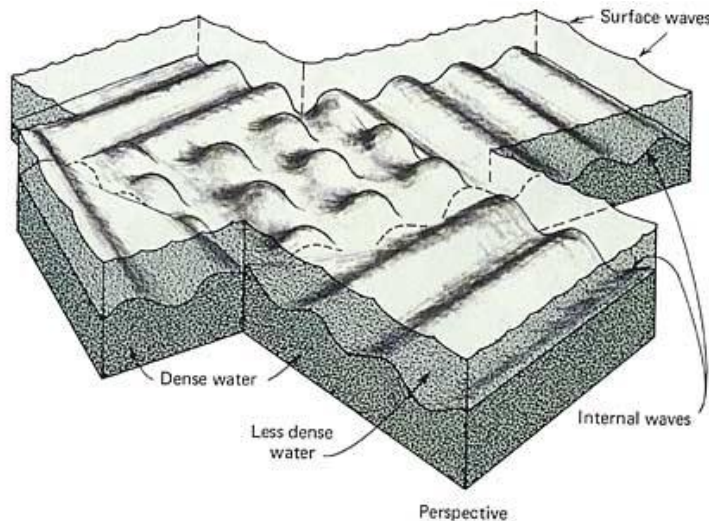
Figuur 16: Inwendige golven bij raakvlak tussen twee lagen water van verschillende dichtheden. De ene heeft een hogere dichtheid (de onderste) dan de andere (de bovenste) ( Oceanography , Gross, p.204).
