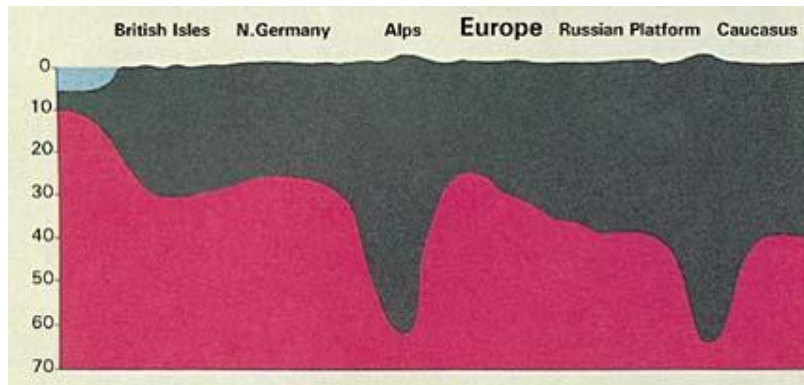
Figuur 8: Schematische doorsnede. De bergen lijken op pinnen en hebben diepe wortelen ingebed in de grond. ( Anatomy of earth , Cailleux, p.220)
