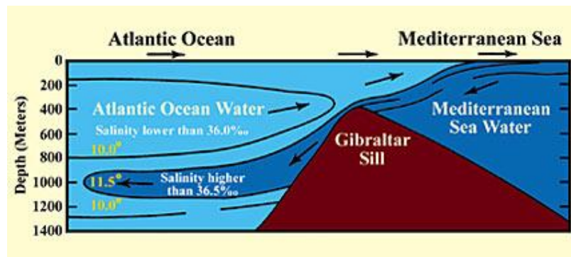
Figuur 13: (De gestabiliseerde toestand van) het Middellandse Zeewater zoals het de Atlantische Oceaan binnenkomt over de rotslaag van Gibraltar. Het heeft zijn eigen kenmerkende temperatuur, zoutgehalte en lage (stof)dichtheid, vanwege de barrière die hen van elkaar onderscheidt. Temperaturen zijn in graden Celsius (°C). ( Marine Geology , Kuenen, p.43).
