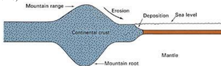
Figuur 9: Een andere illustratie laat zien hoe de bergen een pin-achtige vorm hebben, door hun diepe wortelen. ( Earth Science , Tarbuck en Lutgens, p.158.)
