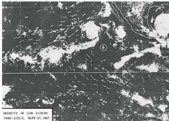
Figuur 17: Satelliet foto toont de wolken, die in de (verzamel)gebieden B, C en D samenkomen. De pijlen geven de windrichting aan. ( The Use of Satellite Pictures in Weather Analysis and Forecasting , Anderson en anderen, p. 188)
