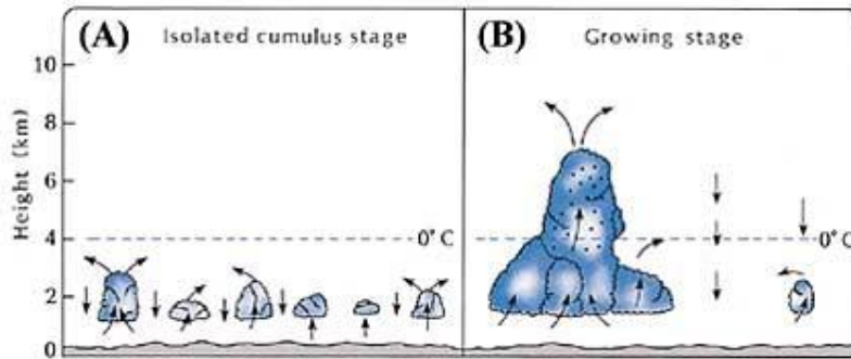
Figuur 19: (A) Geïsoleerde kleine wolk eenheden (cumulus wolken). (B) (Groeï stadium:) Als de kleine wolken samengevoegd worden, neemt de opstijgende lucht binnen de grote wolken toe, dus stapelt de wolk zich op. Waterdruppels worden aangeduid met •. ( The atmosphere , Anthes en anderen, p. 269.)
