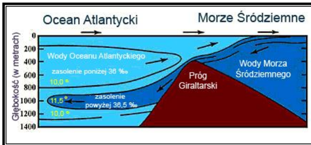
Ryc 13: Wody Morza Śródziemnego wpadające do Atlantyku nad progiem Gibraltarskim zachowują swoje własne ciepło, zasolenie i mniejszą gęstość ze względu na barierę, która je rozdziela. Temperatury podane są w stopniach Celsjusza (°C). (Marine Geology, Kuenen, str. 43, z małymi poprawkami).
