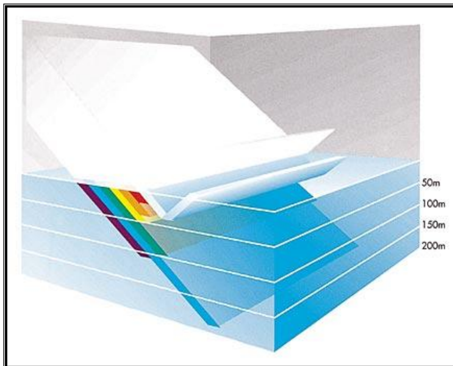
Ryc. 15: Od 3 do 30 procent promieni słonecznych odbija się od powierzchni morza. Potem prawie wszystkie z siedmiu kolorów widma światła są absorbowane, jeden po drugim, w pierwszych 200 metrach, z wyjątkiem światła niebieskiego. (Oceans, Elder and Pernetta, str. 27).
