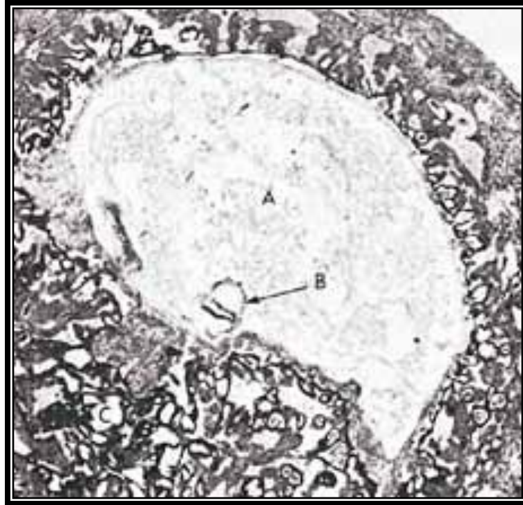
Ryc. 3: Na tej fotografii widzimy zawieszenie embrionu (oznaczony jako B) w fazie alafa (około 15. dnia) w łonie matki. Rzeczywisty rozmiar embrionu to około 0,6mm. ( The Developing Human , Moore, wyd. III, str. 66, from Histology , Leeson and Leeson).
