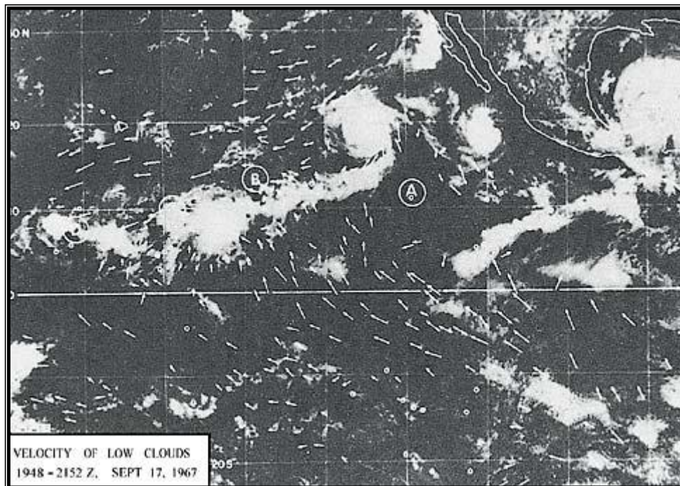
Ryc. 17: Zdjęcie satelitarne, pokazujące przesuwanie się chmur w kierunku obszarów skupiania B, C i D. Strzałki wskazują kierunek wiatru. ( The Use of Satellite Pictures in Weather Analysis and Forecasting, Anderson and others, str. 188 ).
