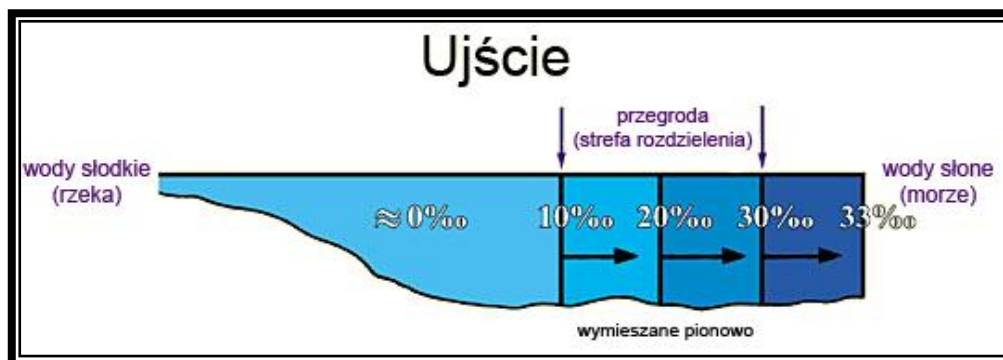
Ryc. 14: Przekrój podłużny pokazujący zasolenie (wyrażone w promilach) w strefie ujścia. Możemy tu zobaczyć przegrodę (strefę rozdzielania) pomiędzy wodami słodkimi a słonymi. (Introductory Oceanography, Thurman, str. 301, z małymi zmianami).
