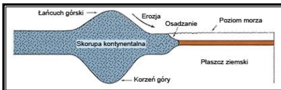
Ryc. 8: Schematyczny przekrój. Góry, jak paliki, mają głębokie korzenie pod ziemią. ( Anatomy of the Earth, Cailleux, str. 220 ).
