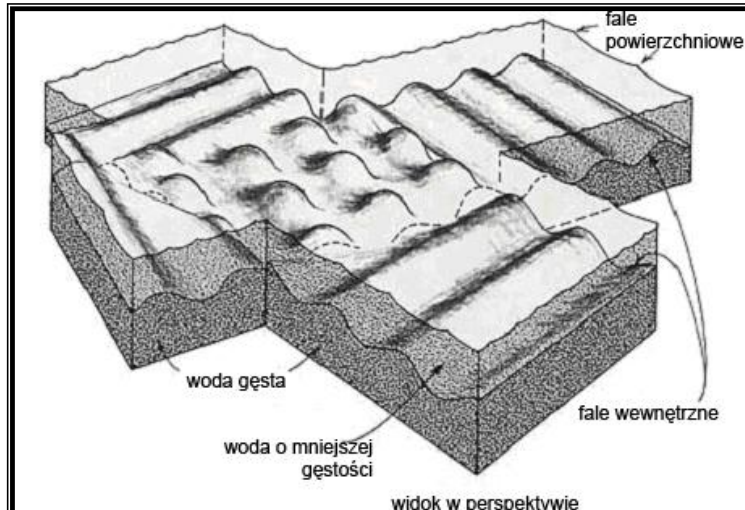
Ryc. 16: Fale wewnętrzne na styku pomiędzy dwiema warstwami wody o różnych gęstościach. Jedna jest gęsta (niższa), druga mniej gęsta (wyższa). (Oceanography, Gross, str. 204).
