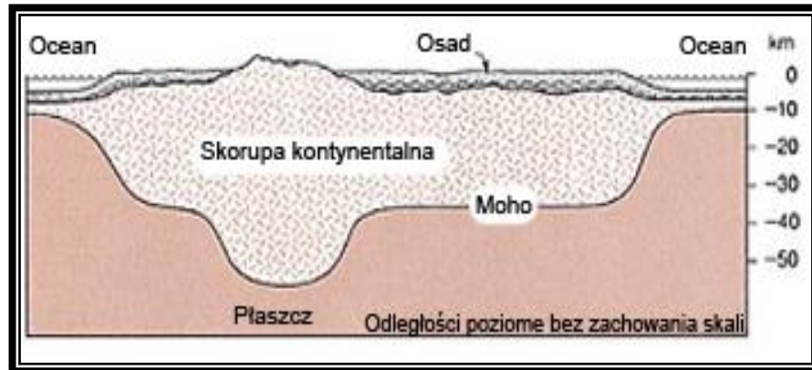
Ryc. 7: Góry mają głębokie korzenie pod powierzchnią ziemi ( Earth, Press and Siever, str.413 ).
